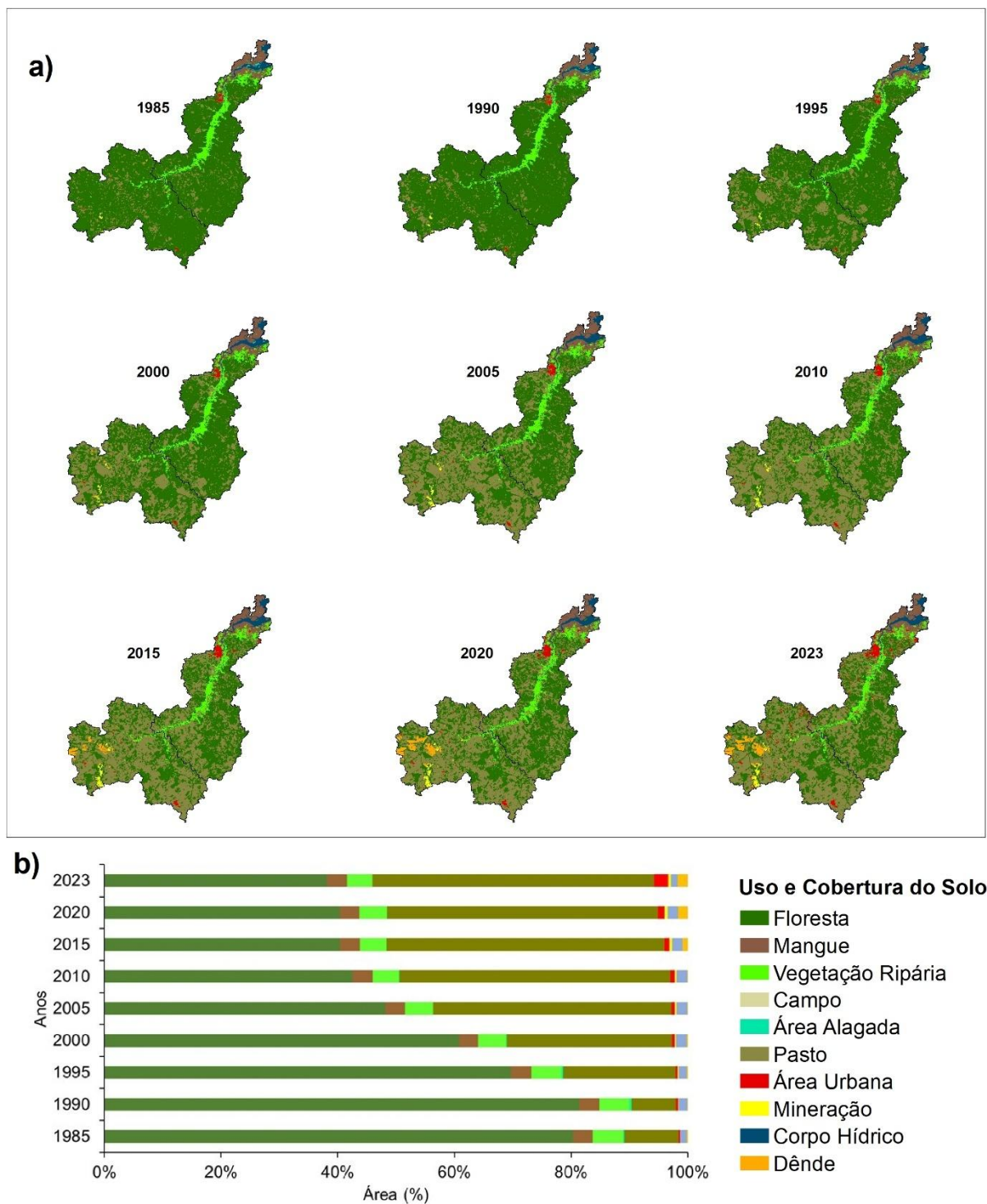
Figura 2. Mudanças espaço-temporais do uso e cobertura do solo (1985-2023): Bacia Hidrográfica do rio Caeté.
