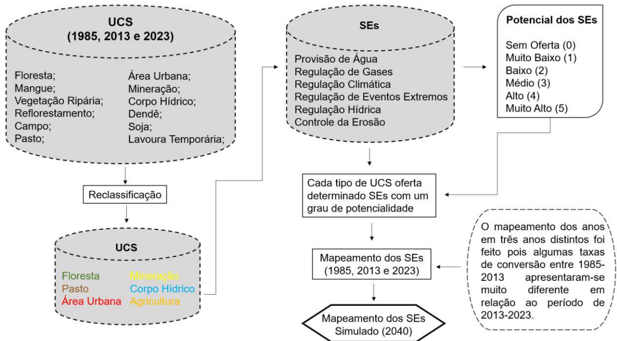
Figura 5. Fluxograma dos procedimentos e etapas metodológicas.
