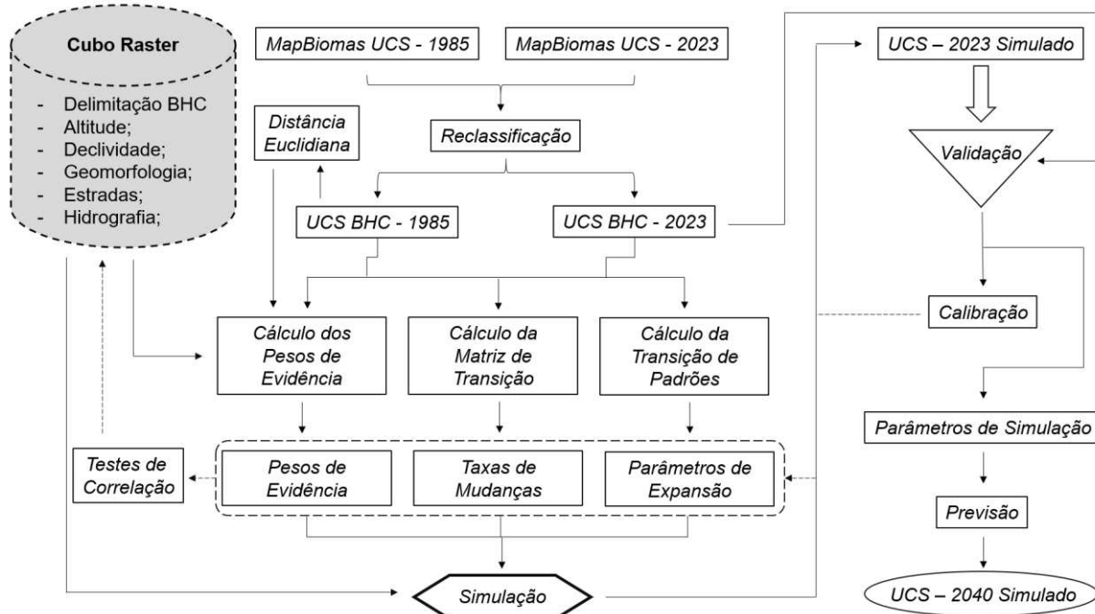
Figura 4. Fluxograma das etapas da modelagem ambiental.
