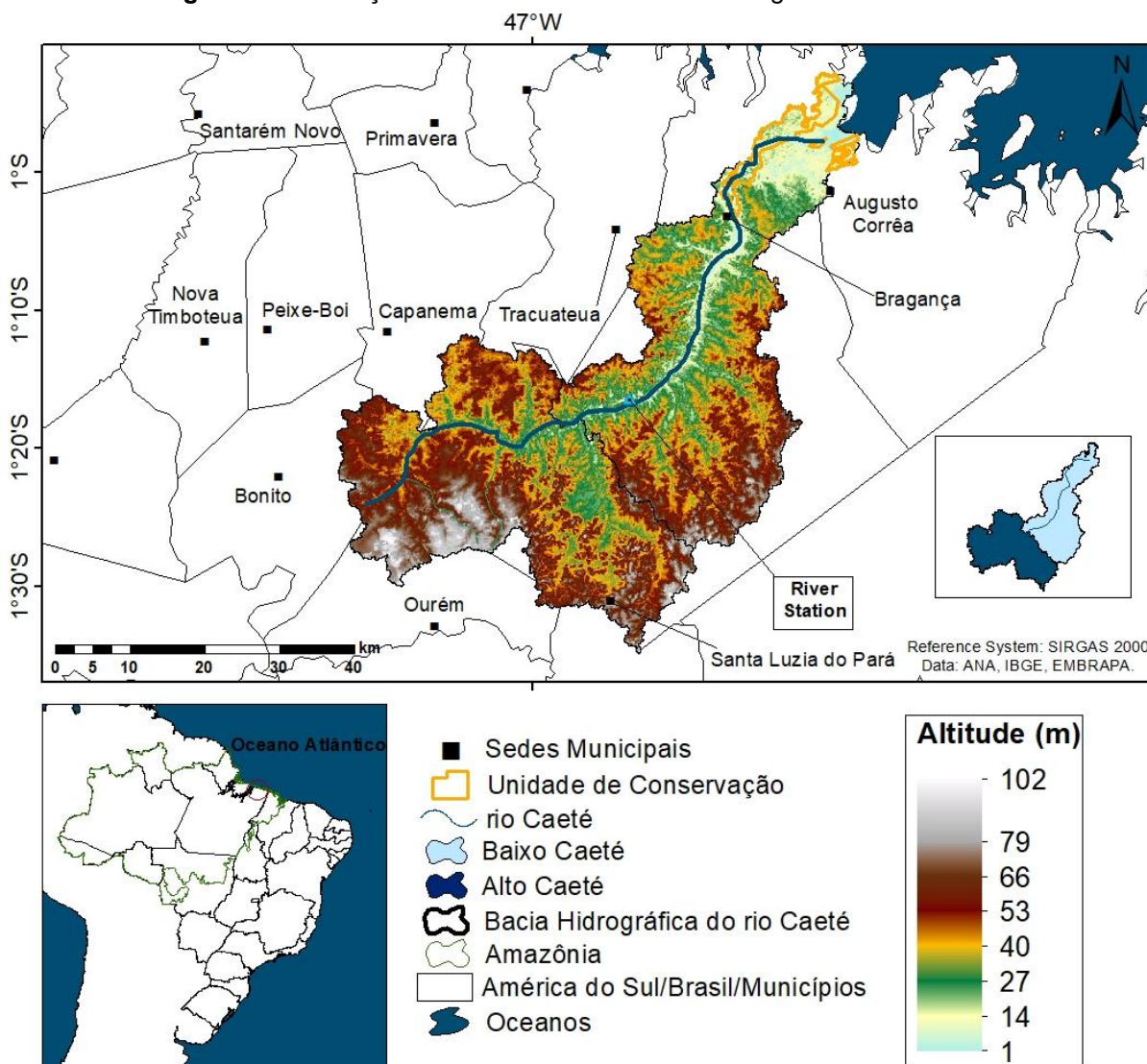
Figura 1. Localização da área de estudo: Bacia Hidrográfica do rio Caeté.
