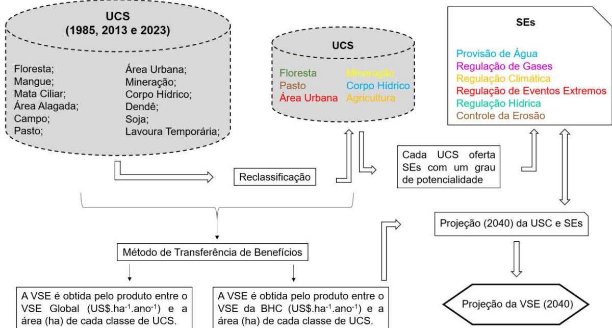
Figura 3. Fluxograma dos procedimentos adotados e etapas metodológicas.
