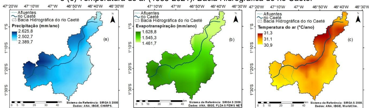
Figura 3. Variabilidade espacial da (a) precipitação (1985-2023), (b) Evapotranspiração (1985-2023) e (c) Temperatura do ar (1985-2021): Bacia Hidrográfica do rio Caeté.
