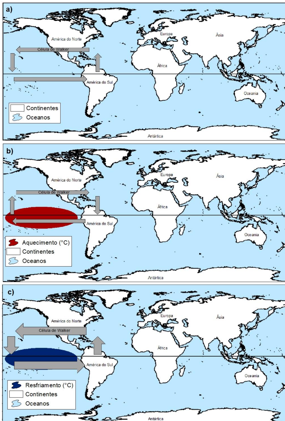
Figura 1. Sistemas de Circulação do Vento na atmosfera: (a) Padrão (Neutro); (b) El Niño; (c) La Niña.
