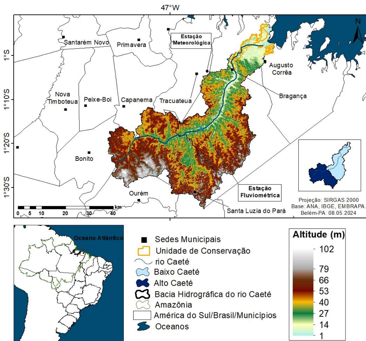
Figura 4. Localização da área de estudo: Bacia Hidrográfica do rio Caeté.
