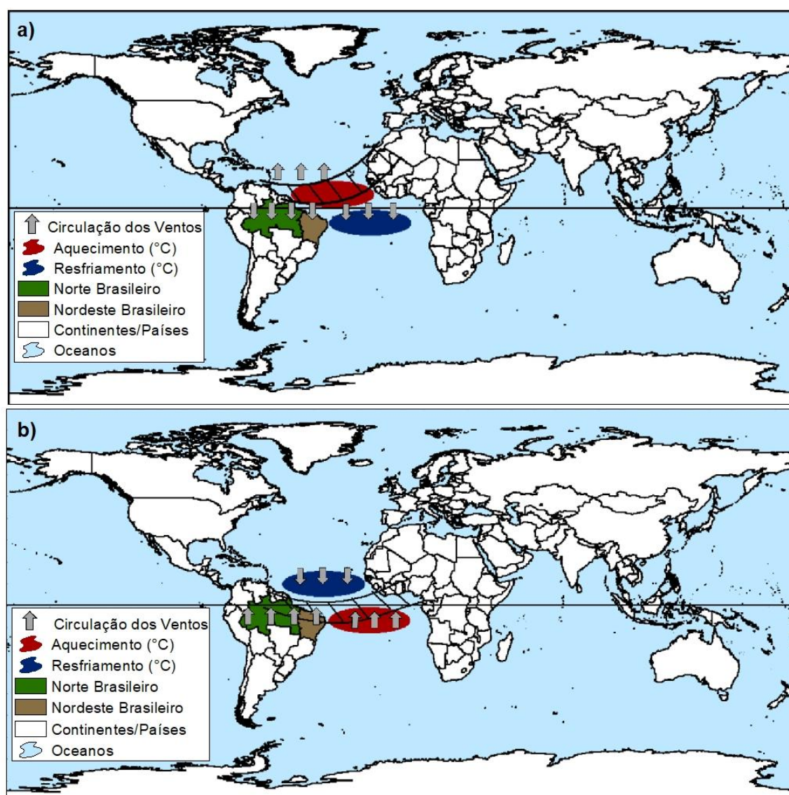
Figura 2. Fenômeno do Dipolo do Atlântico: (a) DA + ; (b) DA - .
