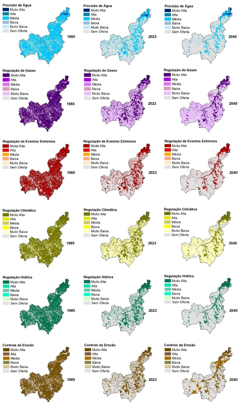
Figura 7. Diagnóstico (1985-2023) e Projeção (2040) da oferta de Serviços Ecossistêmicos da provisão e regulação: Bacia Hidrográfica do rio Caeté.
