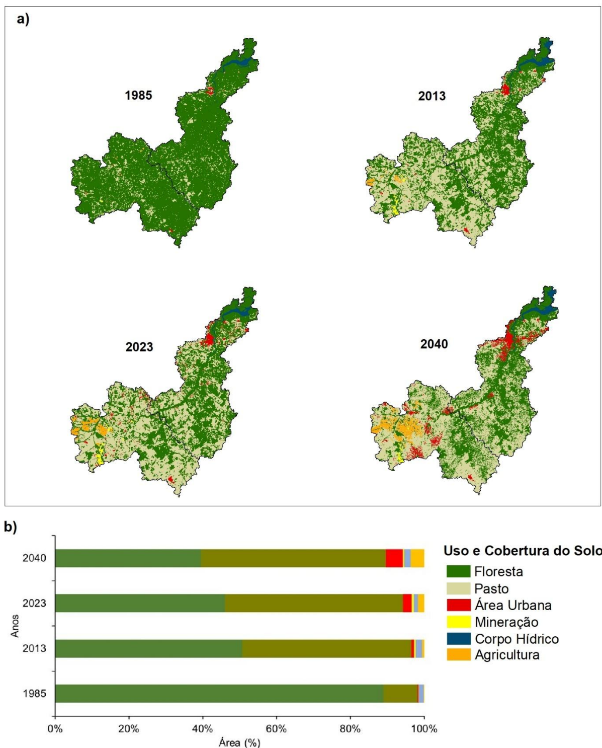
Figura 6. Mudanças espaço-temporais do uso e cobertura do solo reclassificado (1985-2013-2023) e projetado (2040): Bacia Hidrográfica do rio Caeté.
