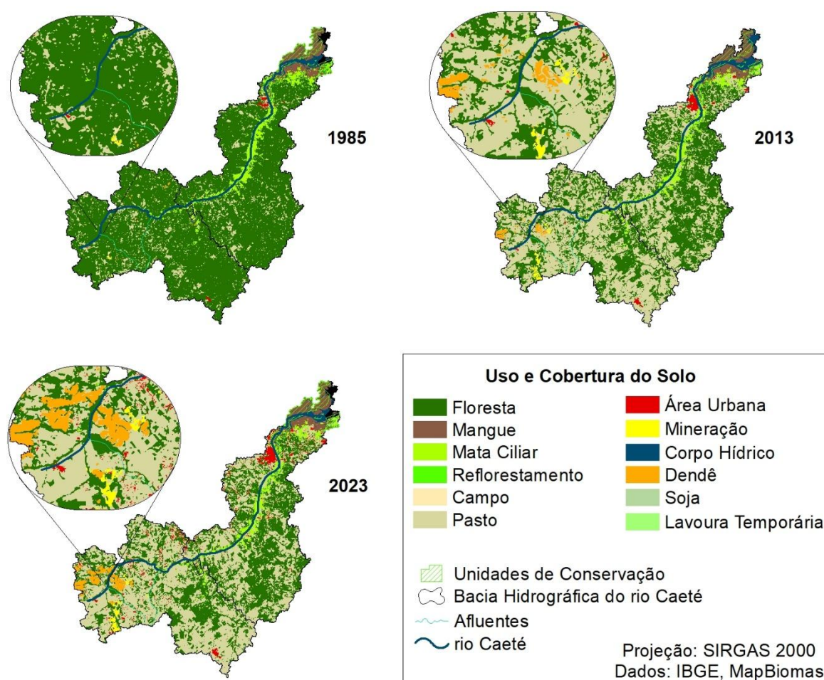
Figura 2. Mudanças do uso e cobertura do solo (1985-2013-2023): Bacia Hidrográfica do rio Caeté.
