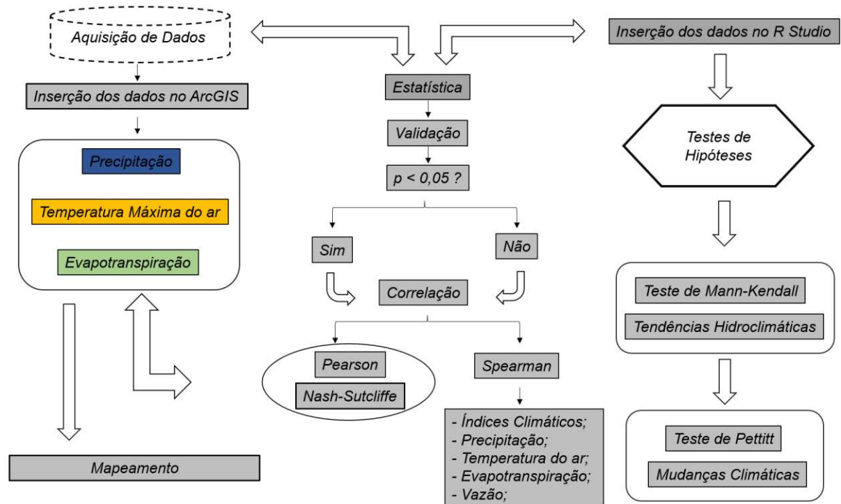
Figura 2. Fluxograma da aquisição e tratamento dos dados.
