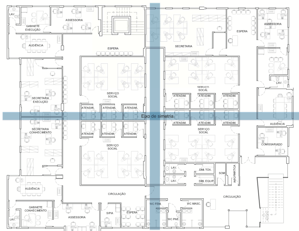
Figura 33 - Planta baixa do pavimento destinado a VIJ TJPA. Fonte: arquivo pessoal.
